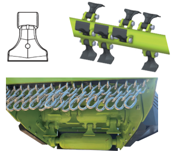
360度揺動刃物 (RTN70)
